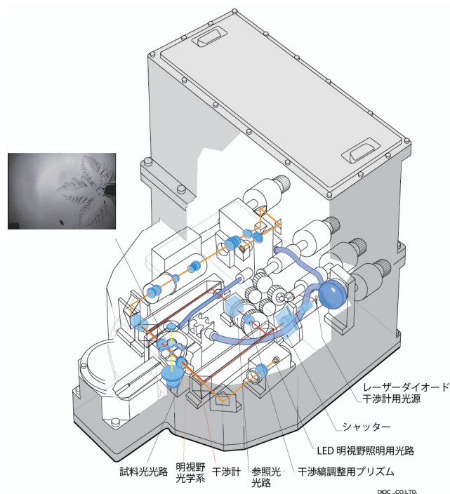
図3 宇宙実験装置 Ice Crystal Cell の透視図。外寸は、25 cm × 30 cm × 21 cm。オリンパス提供。
