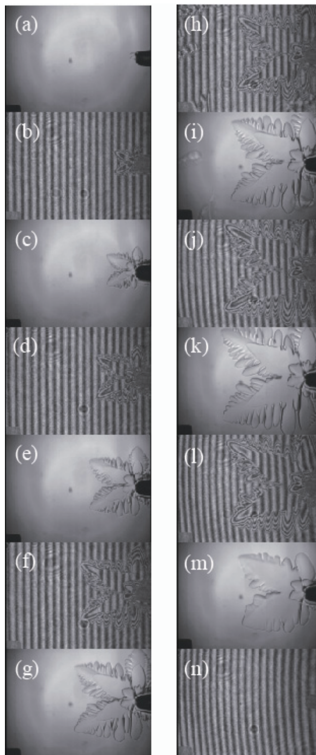
図4 「きぼう」実験で取得された氷結晶成長画像。過冷却度は、 \Delta T=0.4 K。明視野画像と干渉縞画像が交互に切り替わって、地上にダウンリンクされる。各写真の時間間隔は、およそ30秒。各画像サイズは、横幅6.4 mm、高さ4.8 mm。(a)から(h)までは、氷結晶の成長過程、(i)から(n)までは、融解過程を観察している。
