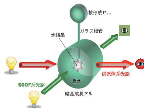
図2 宇宙実験用水結晶成長セルの概念図。
